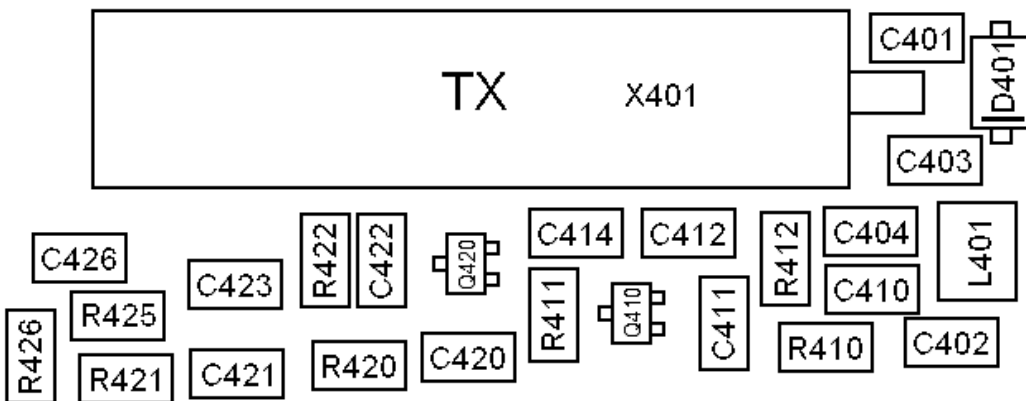
TX VCO
